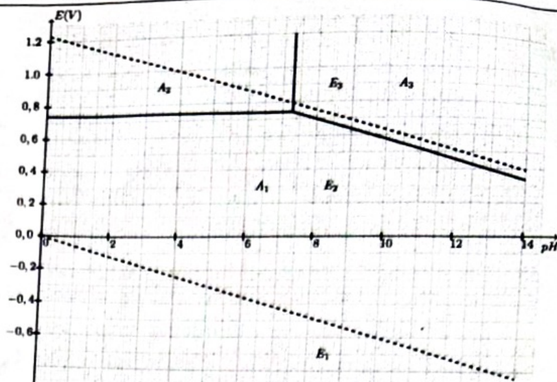
Figure 2 : Diagramme E - pH de l'argent.
