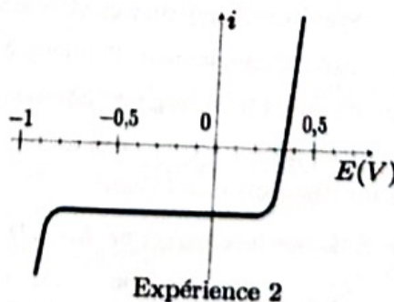
Figure 3 : Courbes intensité-potential enregistrées au cours de l'expérience.
