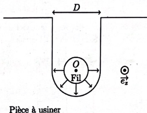
Figure 2-1 : Principe du dispositif de l'électroérosion par fil. Figure 2-2 : Vue de dessus de l'entaille dans la pièce usinée.
