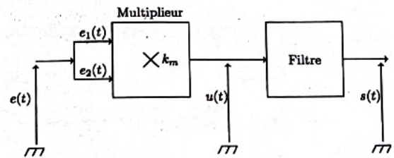
Figure 1-1 : Schéma du doubleur de fréquence.
