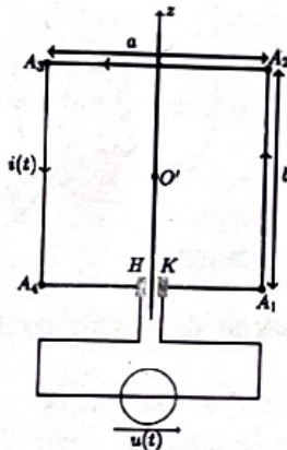
Figure 2-3 : Moteur à courant continu (vue de profil).
