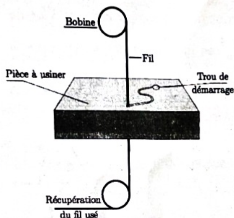
Figure 2-1 : Principe du dispositif de l'électroérosion par fil. Figure 2-2 : Vue de dessus de l'entaille dans la pièce usinée.
