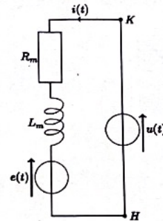
Figure 2-6 : Modèle électrique de l'induit du moteur à courant continu.
